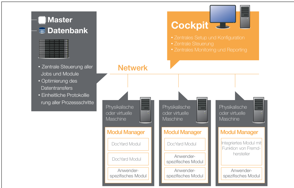
Modulare DocYard-Architektur
